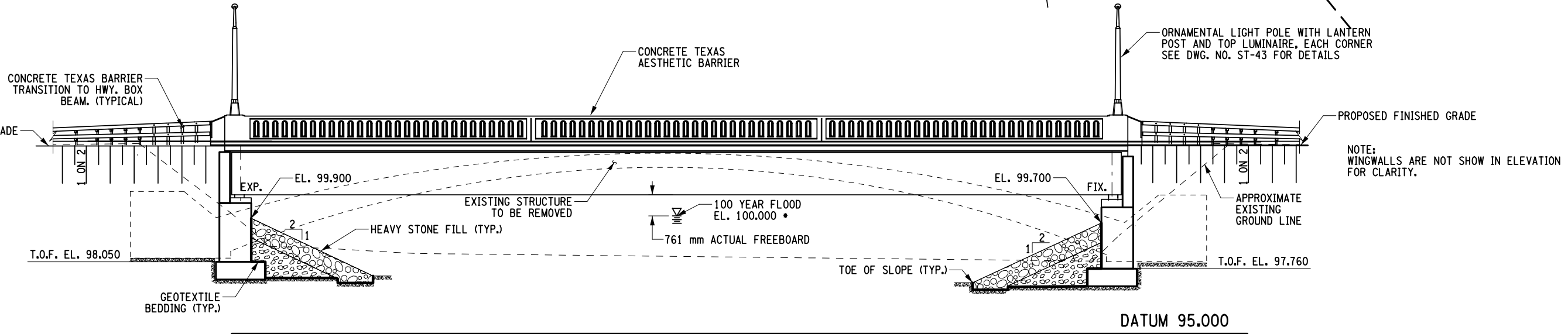
ELEVATION A-A
